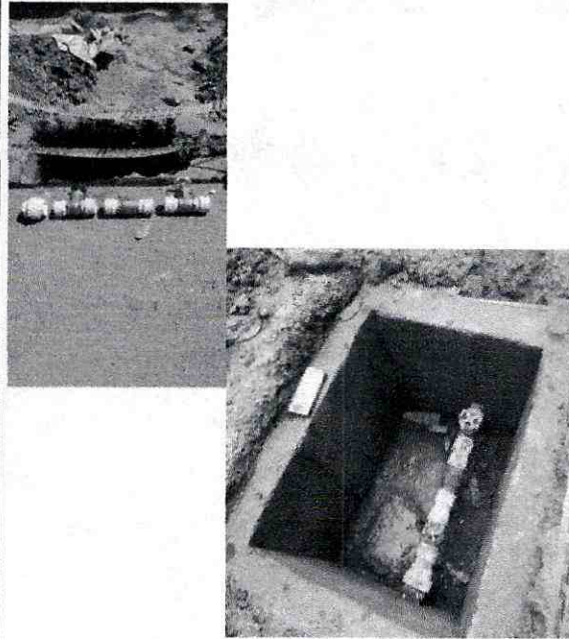
NP12 Suministro e instalación de sistema bypass
