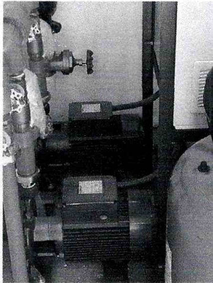
NP11 Sistema bombeo (Incluye 2 motobombas de 4HP, Hidroflow)
