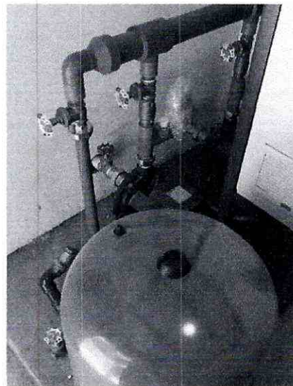
NP12 Suministro e instalación de sistema bypass
