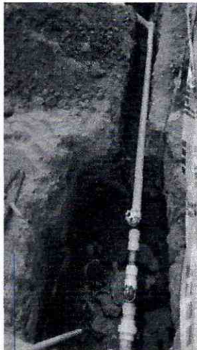
6.5 Suministro e instalación de tubería de 3"
