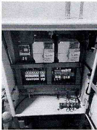
NP09 Sistema de automatización y control del sistema de bombeo presurizado a la red
