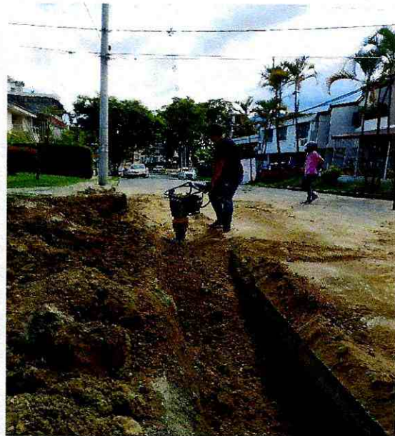
Instalacion de la tubería de 12" Pulgadas presion RDE 21 y llenos en material de recebo compactado mecanimanete para el mejoramiento de la red de conduccion entre el tanque la 30 y el tanque de piedrapintada.
