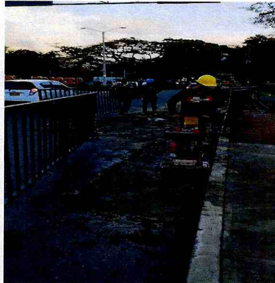
Instalación de la poli sombra para el cerramiento de las excavaciones en el sector y suministro de recebo cemento para mejorar el lleno y nivelar con el pavimento sobre la carrera 5 con calle 43
