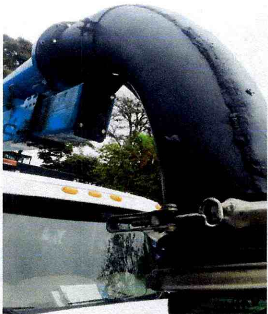
FIGURA 17. INSTALACION DE CODO DE SUCCION CON TORNILLERIA Y SELLOS
