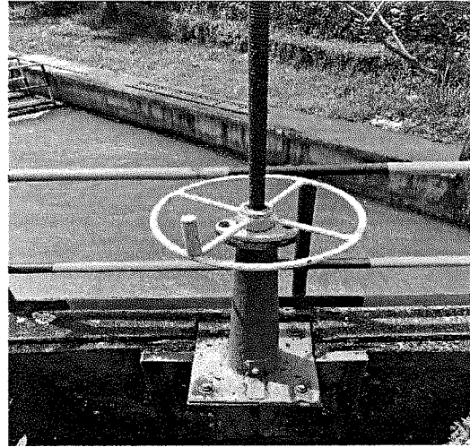
Figura 2. Compuerta de entrada 7 línea 3 reparada.
