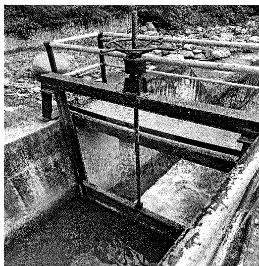
Figura 4. Compuerta del canal de descole(desarenadora) reparada.
