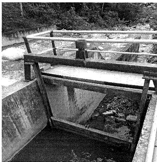
Figura 3. Compuerta del canal de descole(desarenadora) sin espigo y volante.
