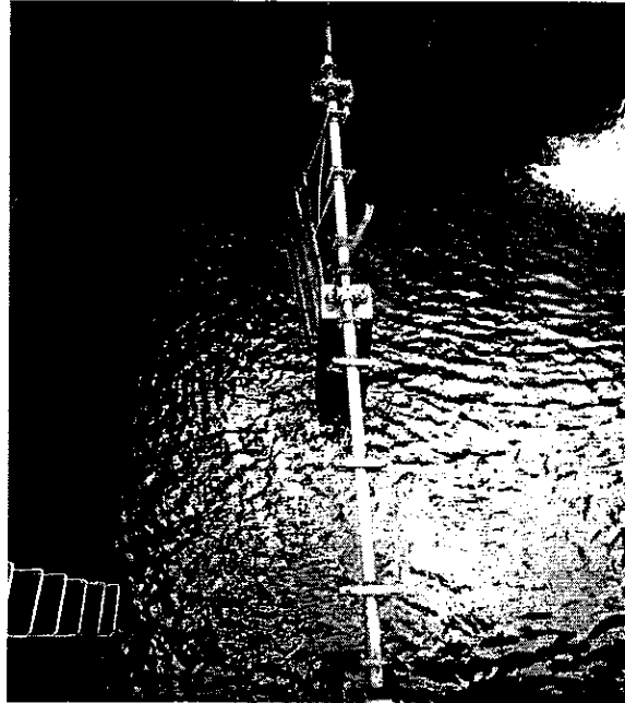
Figura 3. Agitadores floculación horizontal.
