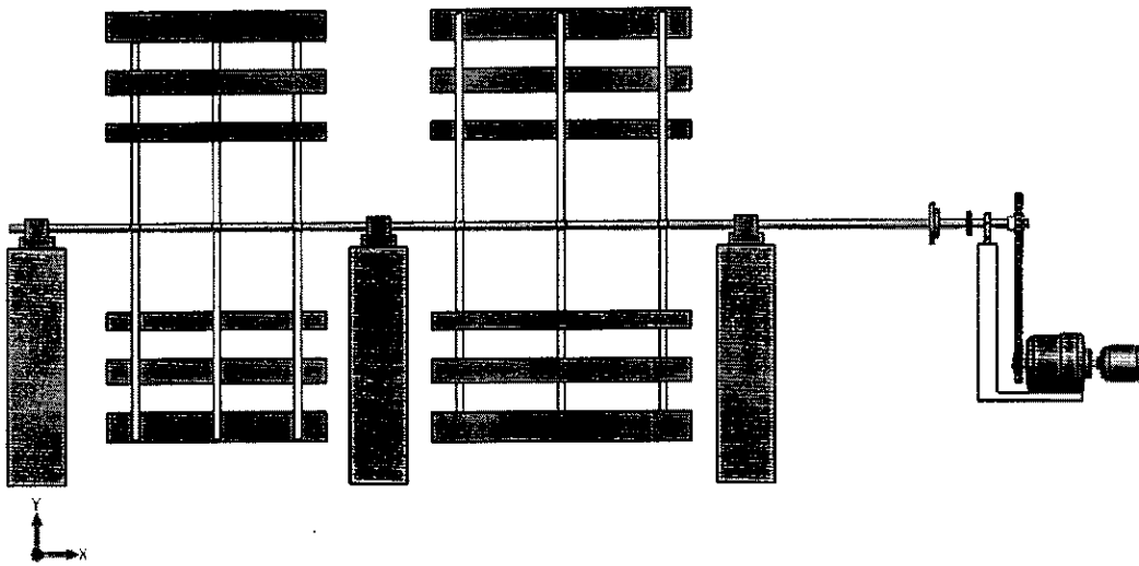
Figura 4. Sistema de floculación horizontal.
