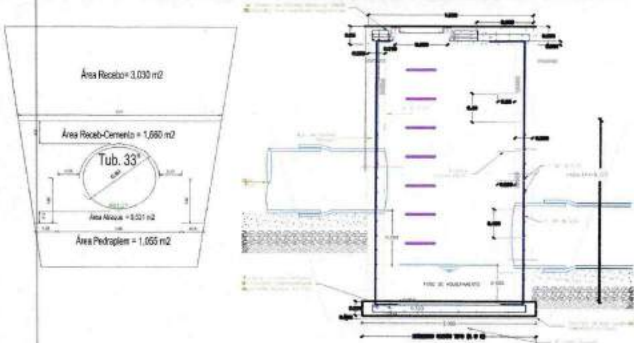
POZO DE INSPECCIÓN Ø1.50m CL/PT/1AM 18/04/2021/DC/AT
