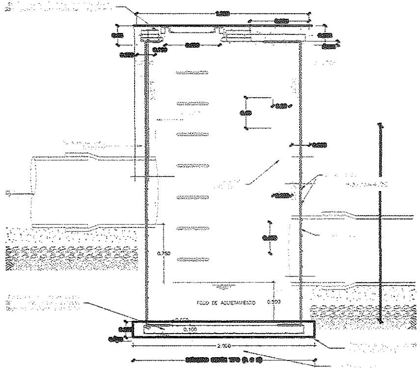
POZO DE INSPECCIÓN Ø1.50m SECCION TRANSVERSAL
