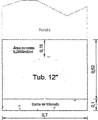
ATRAQUE TUBERÍA RED PRINCIPAL 12"
