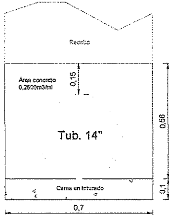
ATRAQUE TUBERÍA RED PRINCIPAL 14"
