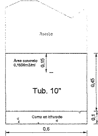
ATRAQUE TUBERÍA SUMIDERO
