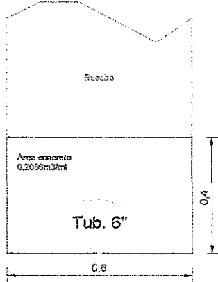
ATRAQUE TUBERÍA DOMICILIARIA 6"
