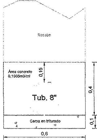
ATRAQUE TUBERÍA RED PRINCIPAL 8"
