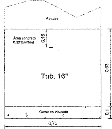
ATRAQUE TUBERÍA RED PRINCIPAL 16"
