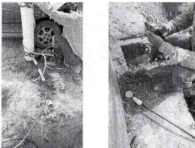
Ilustración 13. Prueba hidrostática Alaska.
