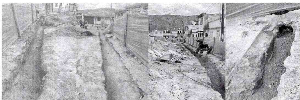
Ilustración 12. Lleno y compactado con recebo Alaska.
