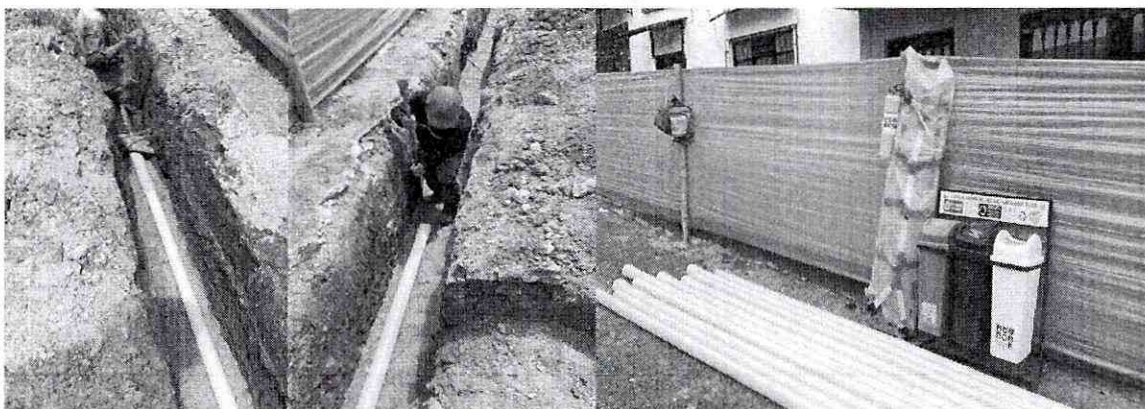
Ilustración 10. Instalación tubería 3"
