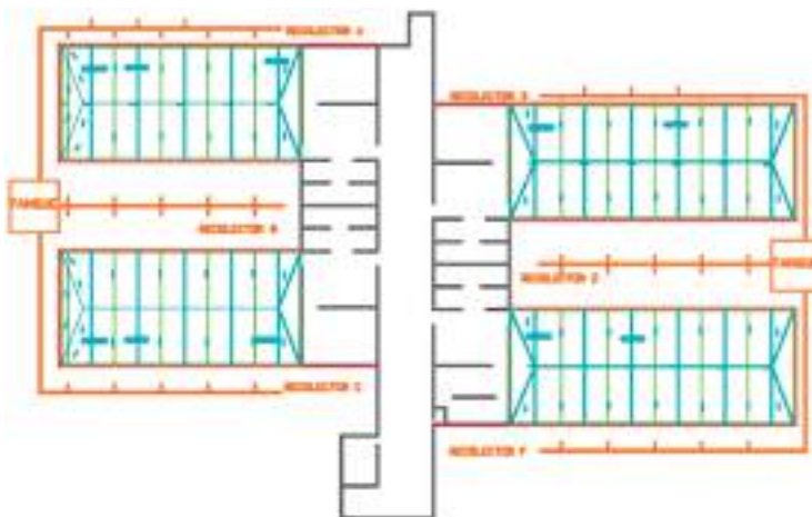
Figura 3. Sistema de recolección de agua lluvia del edificio BACAD 1 de la ESMIC. Fuente: Original de los autores.
