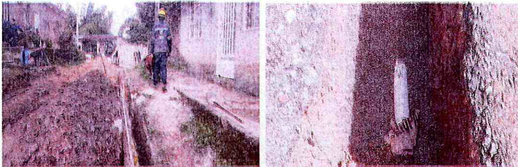
Instalación de tubería red principal de acueducto
