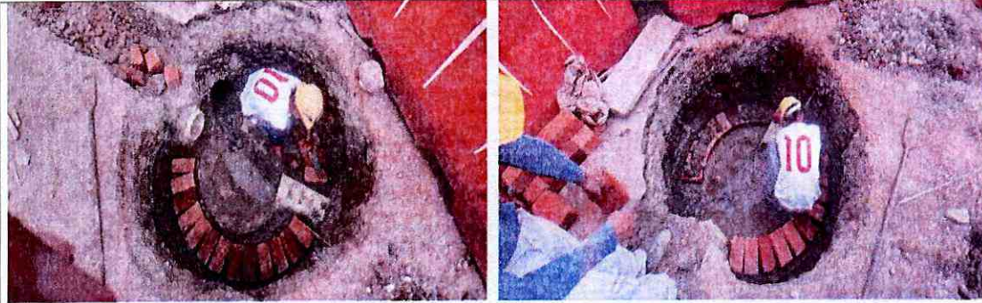
Elaboración de pozo de inspección aguas negras.
