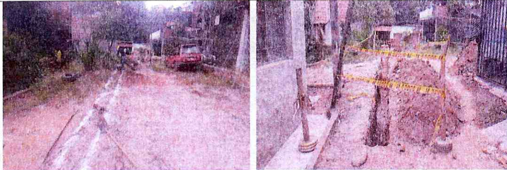
Instalación de tubería red principal de acueducto.
