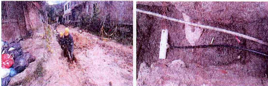
Excavación para tubería red principal de acueducto, instalación de collarines y acometidas red acueducto.
