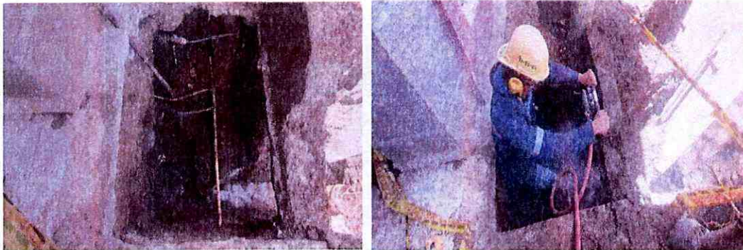
Excavación para caja de acometida alcantarillado.
