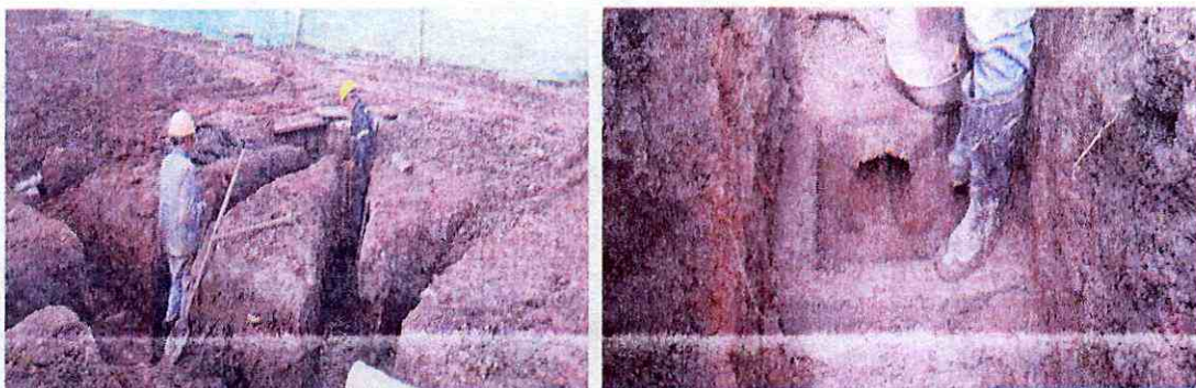
Excavación para tubería sumideros aguas lluvias, fundición caja de transición de tubería de cemento a PVC.
