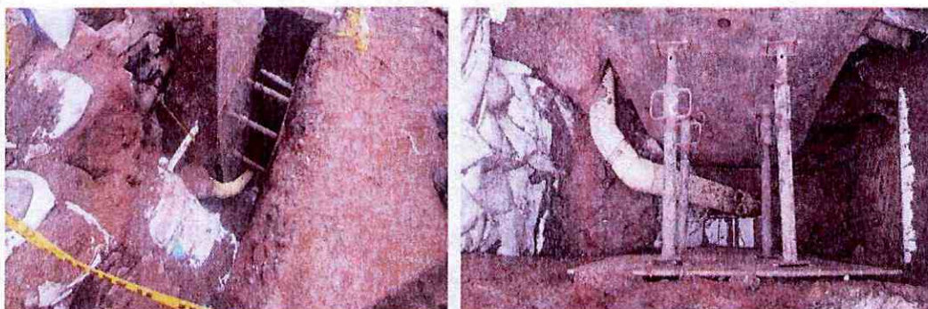
instalación de tubería acometida alcantarillado.
