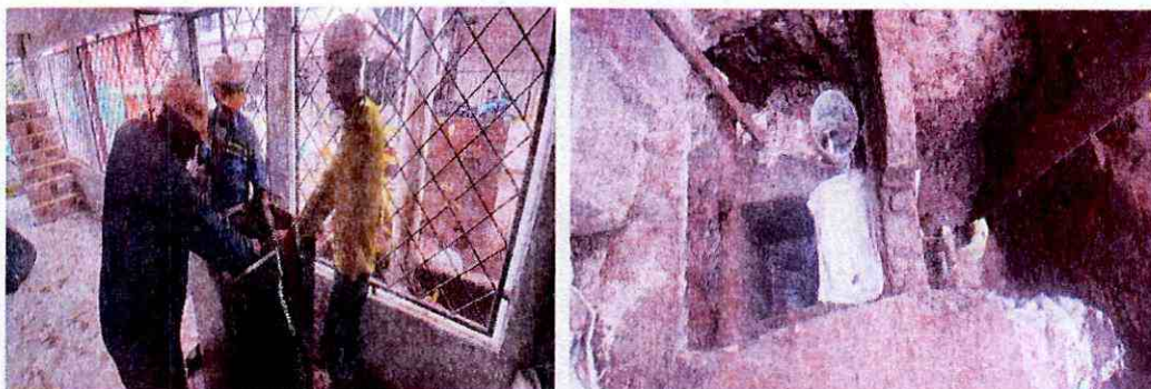
Elaboración de caja de inspección aguas negras.
