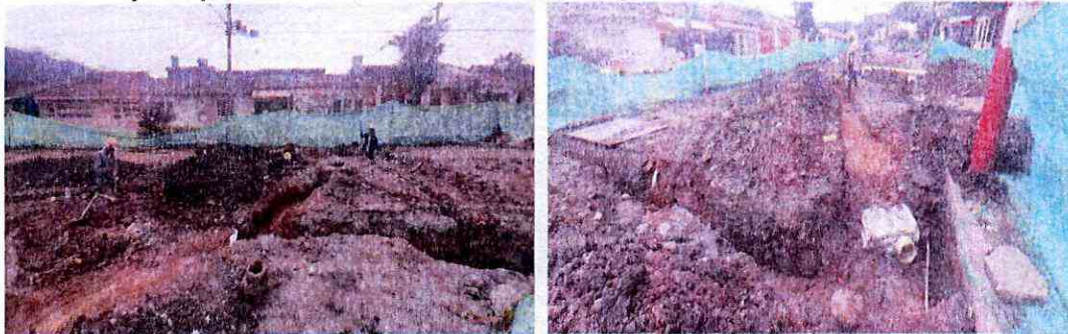
Lleno y compactación de recebo en excavación para tubería sumideros aguas lluvias, instalación de tubería sumideros aguas lluvias.
