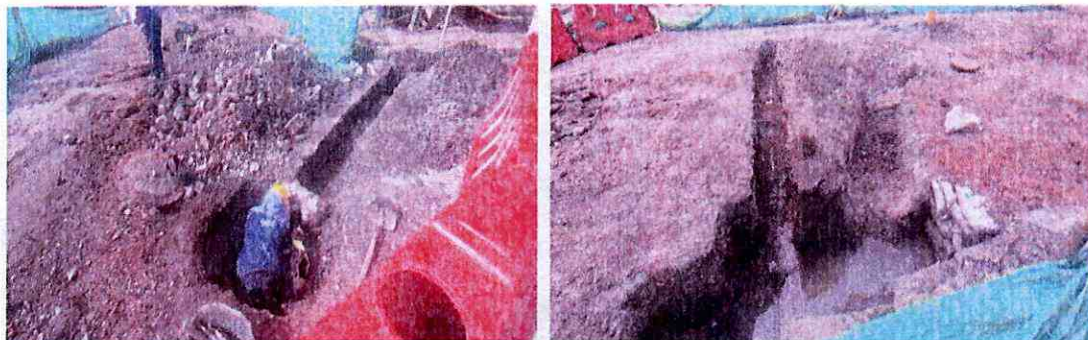
Instalación y recubrimiento de tubería PVC para sumideros, excavación para encontrar tubería para empalme.
