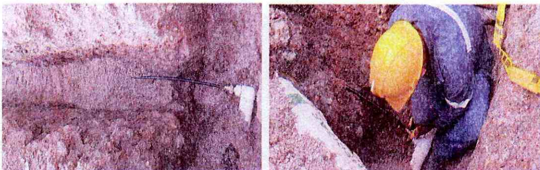
Lleno con arena para acometidas acueducto, instalación de collarines y acometidas red acueducto.
