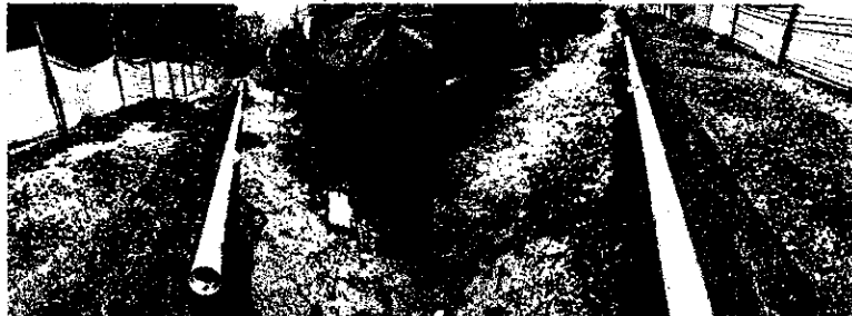
Nivelación de tubería por parte del equipo de topografía con participación de la interventoría
