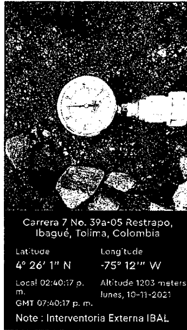
Ilustración 46. Prueba Hidrostática
