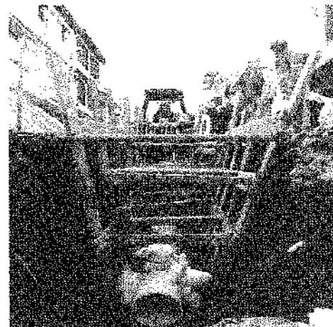
ENTIBADO DE ZANJA
