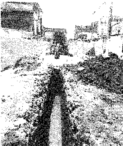
Proceso de excavación e instalación de Tubería Red Principal
