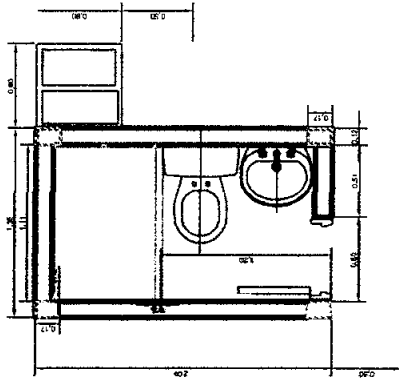
PLANTA UNIDAD SANITARIA
