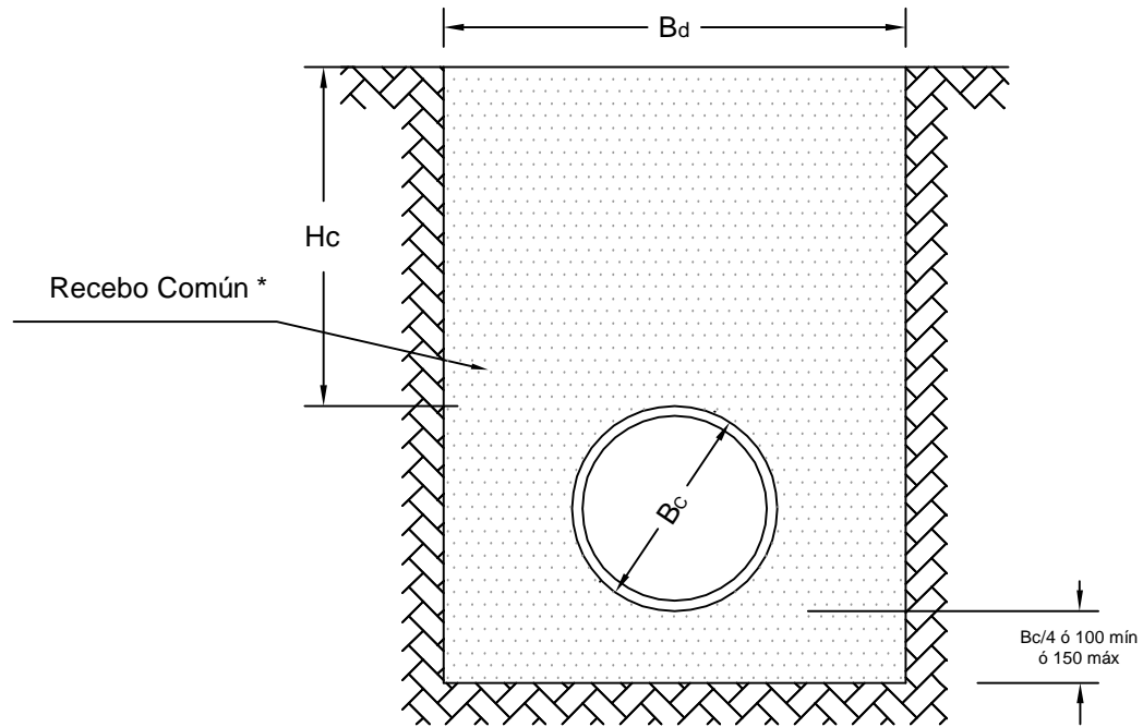
Modelo de Cimentación para tuberías bajo zonas sin tráfico vehicular
