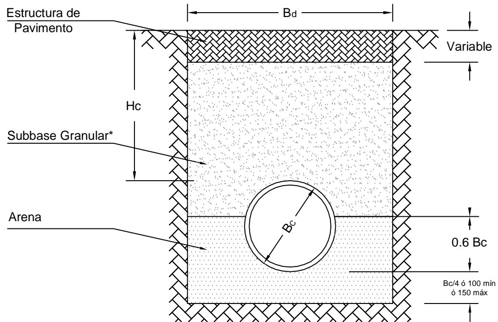
Modelo de Cimentación para tuberías bajo vías, en tramos donde se encuentren suelos no adecuados para fundación de las tuberías.
