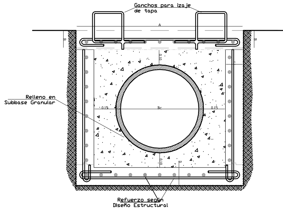
DETALLE DE CARCAMO A, B, C, D: Dimensiones del Cárcamo (Según Diseño Estructural)
