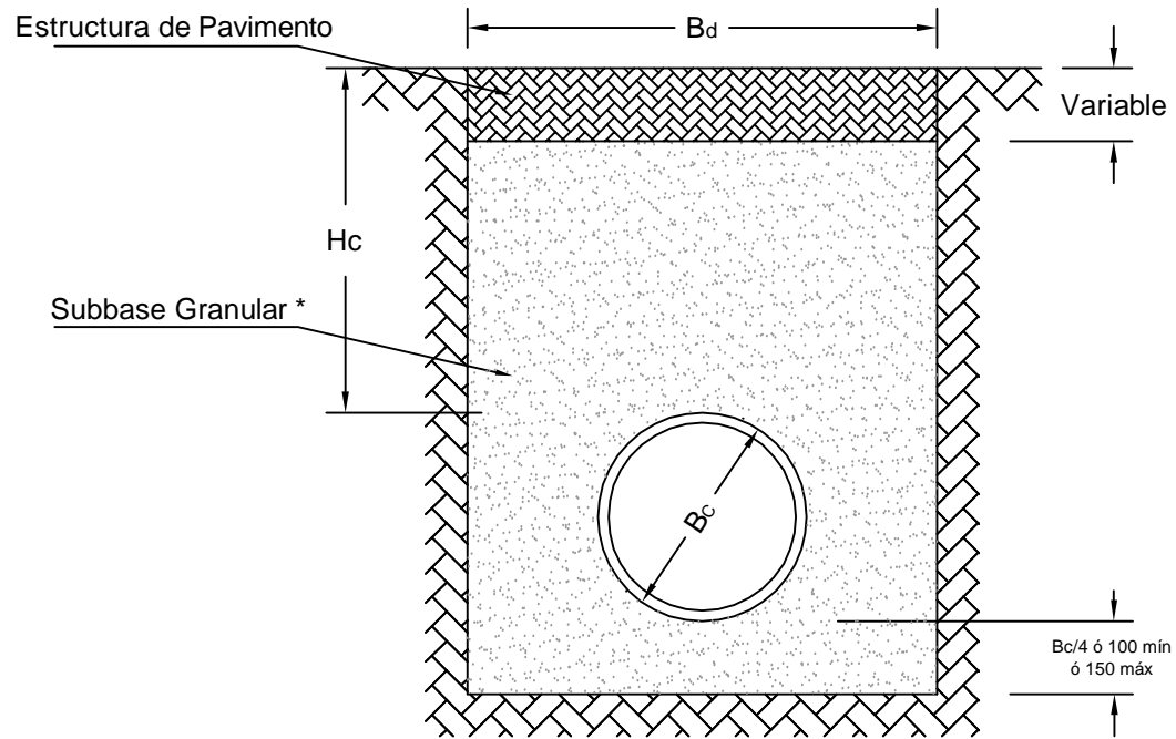
Modelo de Cimentación para tuberías bajo zonas de tráfico vehicular
